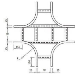
LIEQX (I/R TYPE) LZEQX (Z TYPE) LOEQX (O/R TYPE) 90DEG EQUAL CROSS
