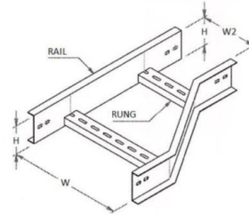
LILRR (I/R TYPE) LZLRR (Z TYPE) LOLRR (O/R TYPE) LEFT-HAND REDUCER
