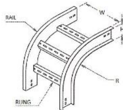
LIRO2 (I/R TYPE) LZRO2 (Z TYPE) LORO2 (O/R TYPE) 90DEG OUTSIDE RISER
