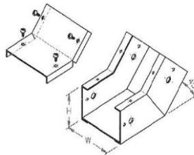
TKI1R 45DEG INSIDE RISER
